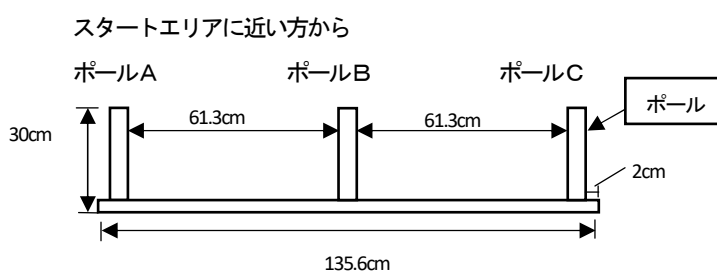
図2. 3本のポールとポール台
